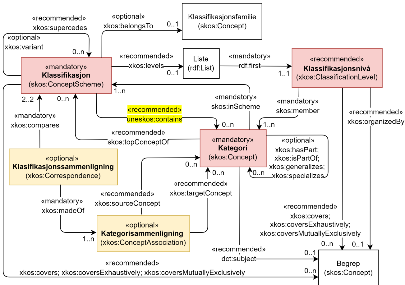
Figur 5. Forenklet modell for XKOS-AP-NO, med alle klasser.
